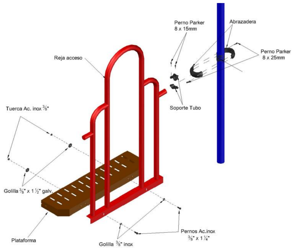
Escala a Reja de Acceso
