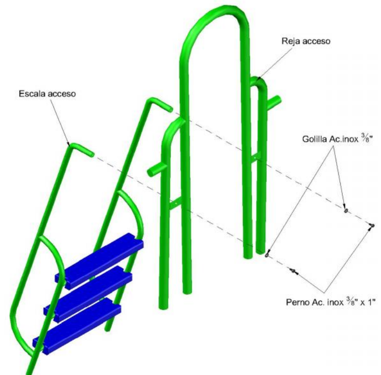
Trepador Vertical a Reja Cobra
