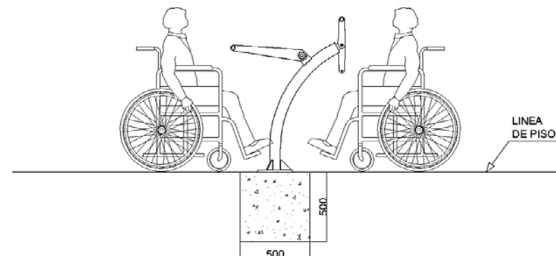
ELEVACION FRONTAL
